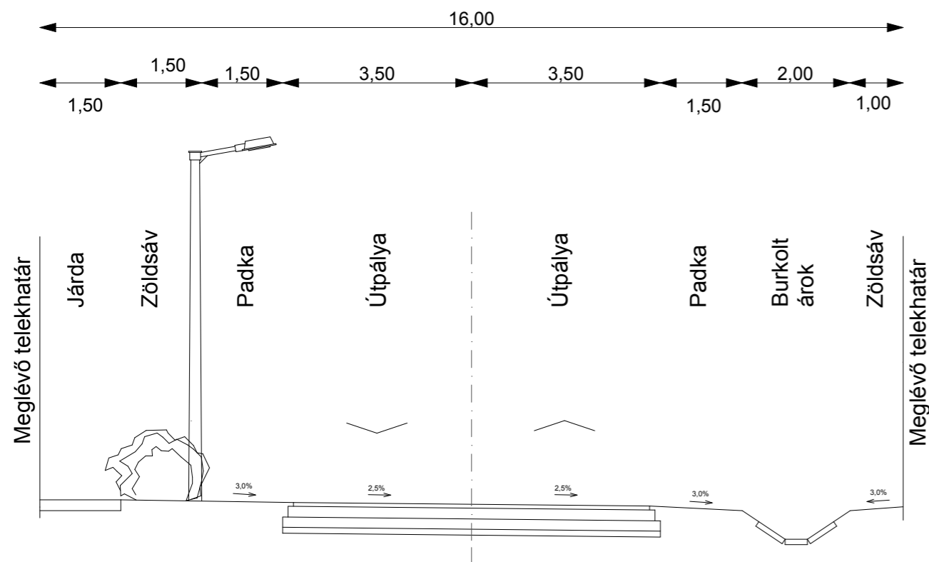
16,0 m széles általános gazdasági területet kiszolgáló út általános mintakeresztmetszele
