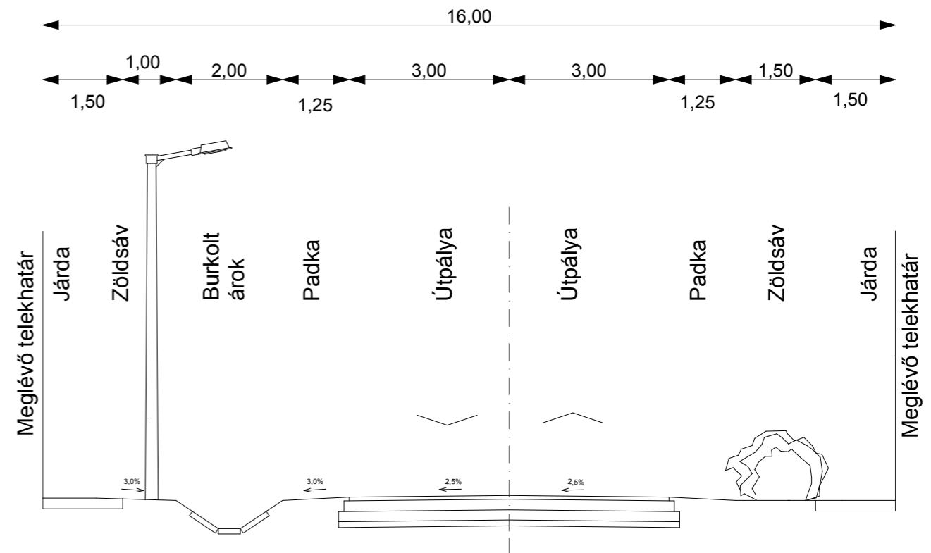
16,0 m széles tervezett lakó utca általános mintakeresztmetszele
