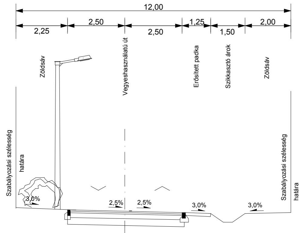
12,00 m széles kiszolgáló út általános mintakeresztmetszele (Vegyeshasználatú út)
